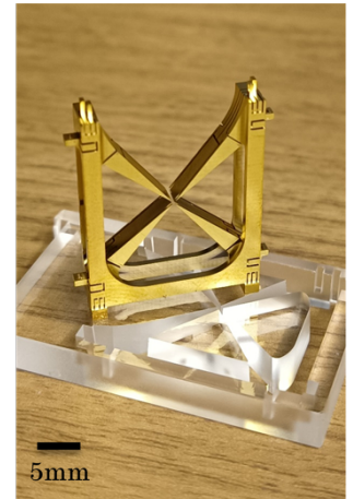
図 1. ガラス基板上に乗せた、金メッキを施した 3D プリント製のイオン・トラップ
